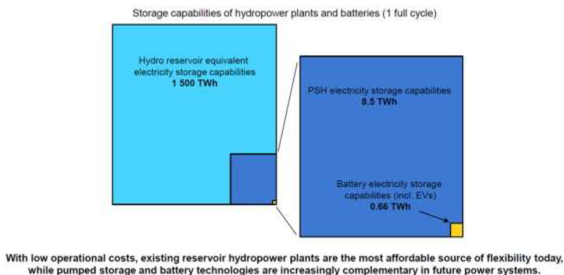
Figura 3 – Armazenamento global de energia elétrica por hidroelétricas em 2020 (IEA)
